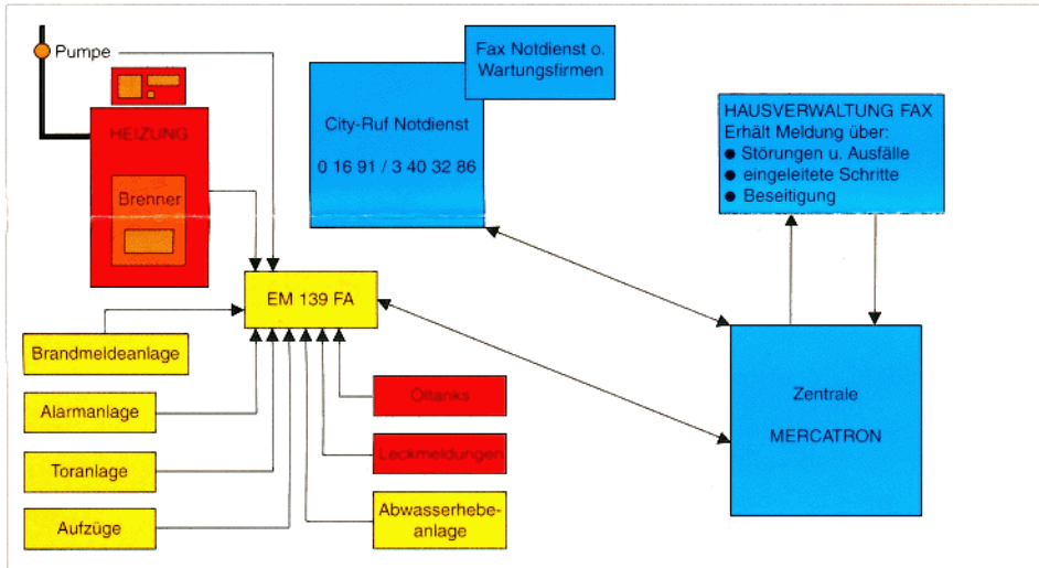
Schema des Mercatron-Fernüberwachungssystems. Eine von vielen Varianten.
