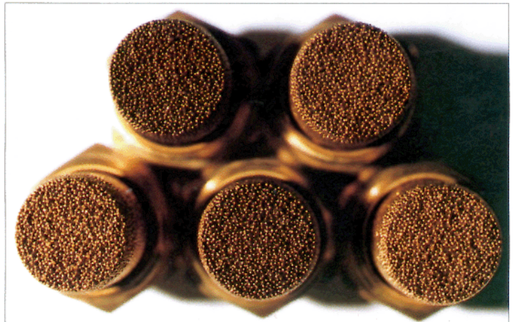
Ölbrennerdüsen nach 700stündigem Test. Links ohne Additiv HEL Guard, rechts mit Additiv HEL Guard. Der Unterschied ist frappant und macht jeden weiteren Kommentar überflüssig.
